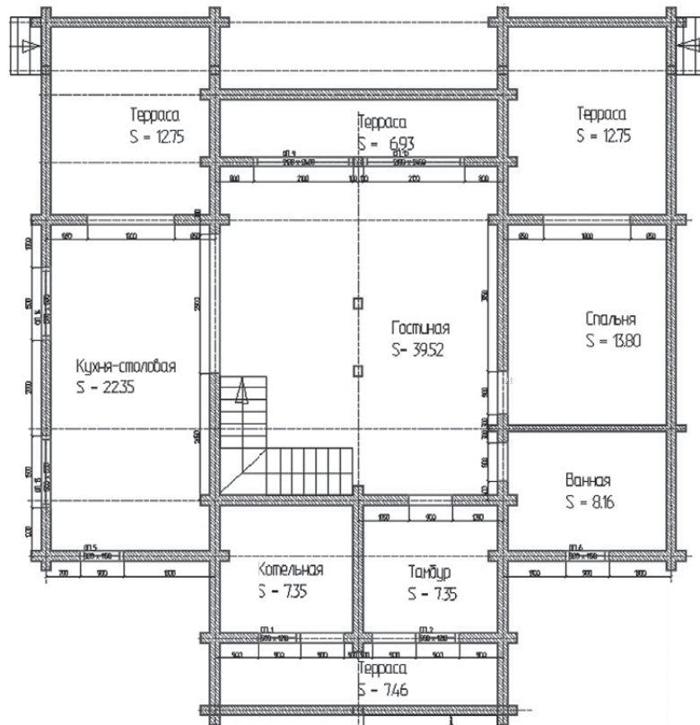
План 1 этажа
