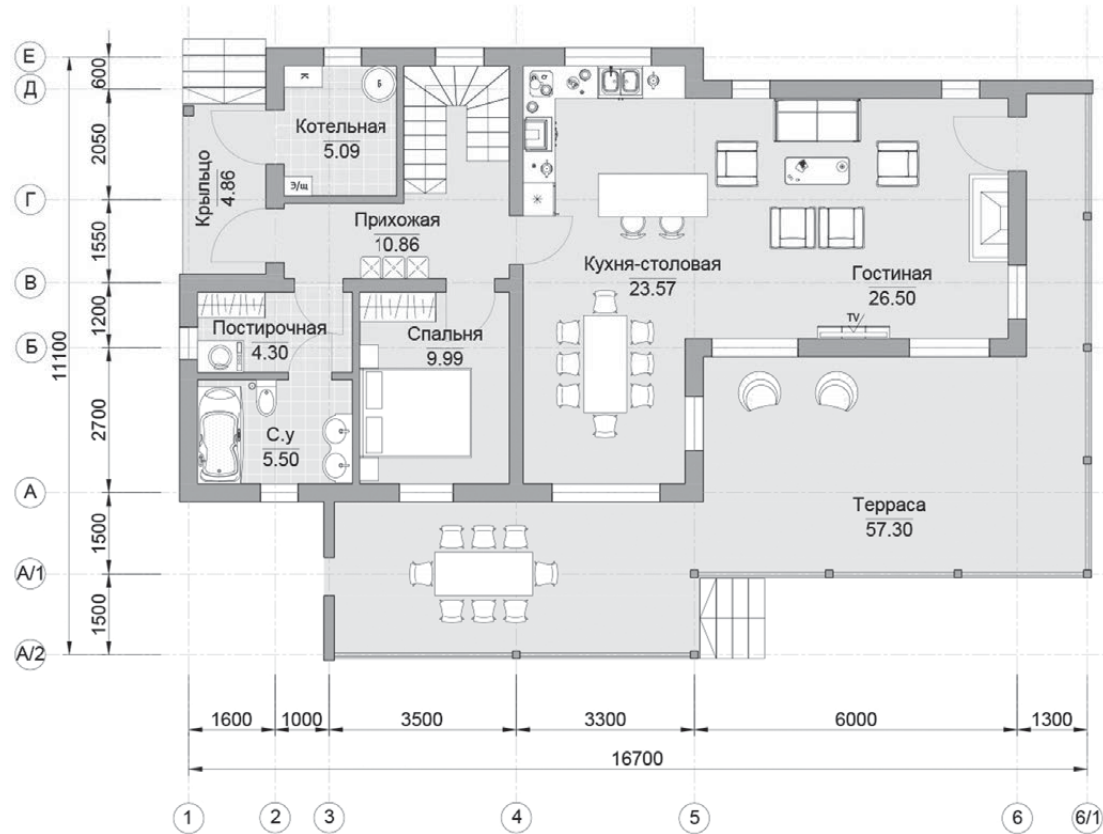
План 1 этажа
