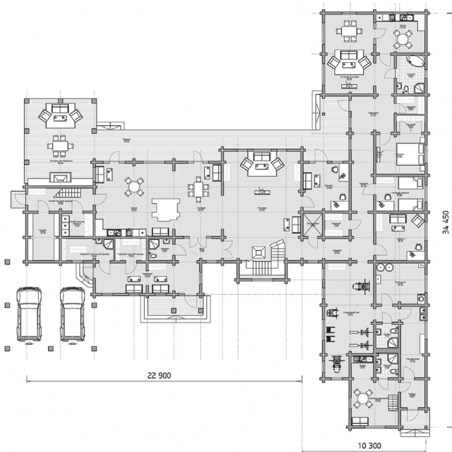
План 1 этажа
