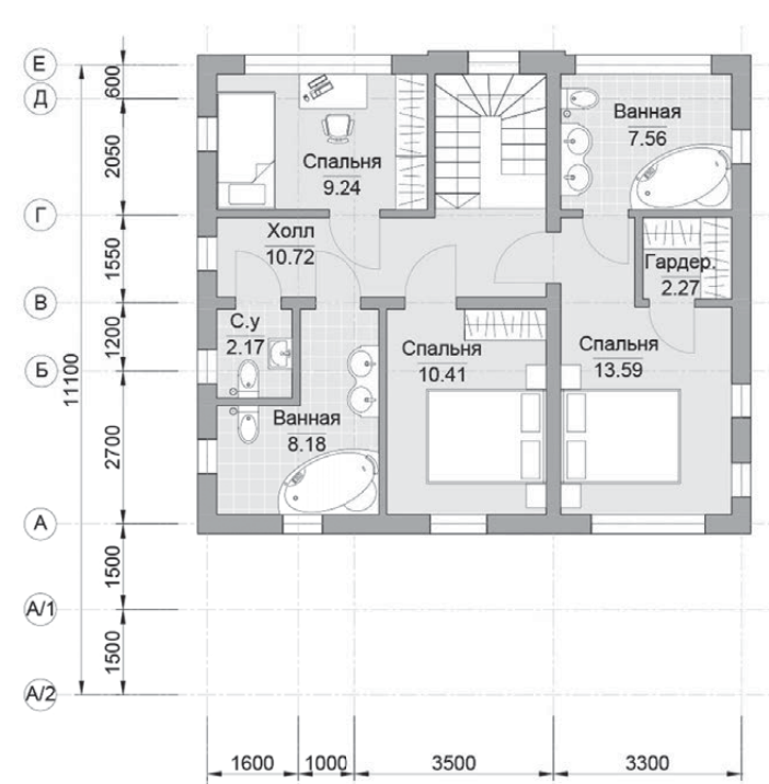
План 2 этажа
