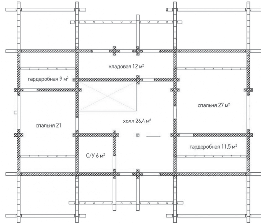
План 2 этажа
