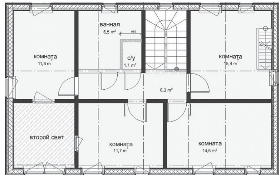
План 2 этажа
