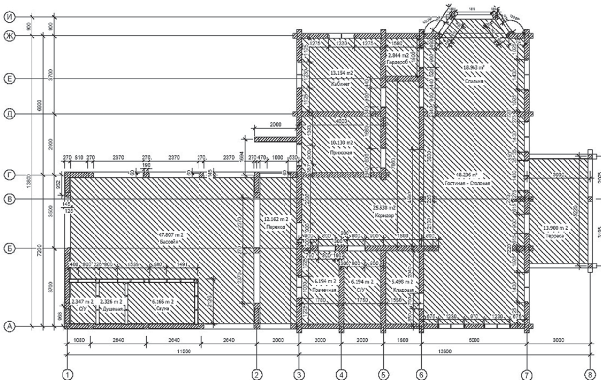
План 1 этажа
