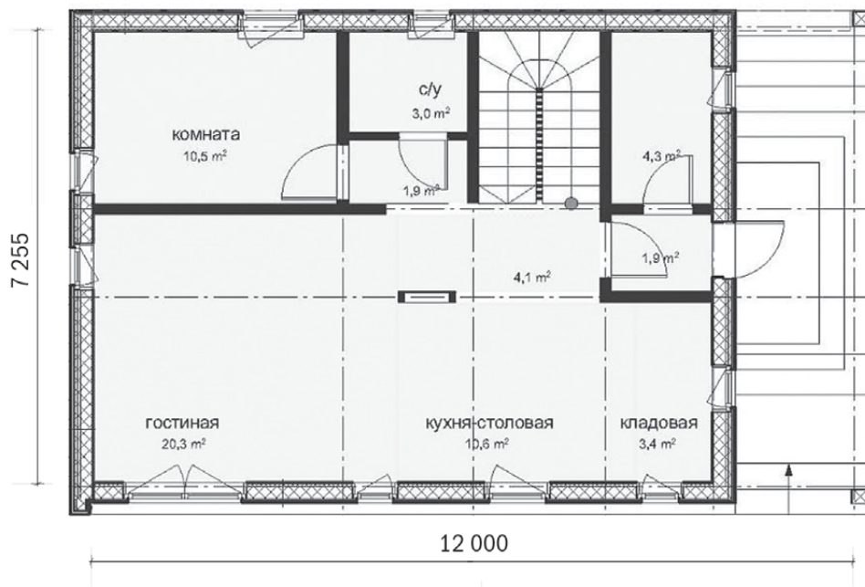
План 1 этажа
