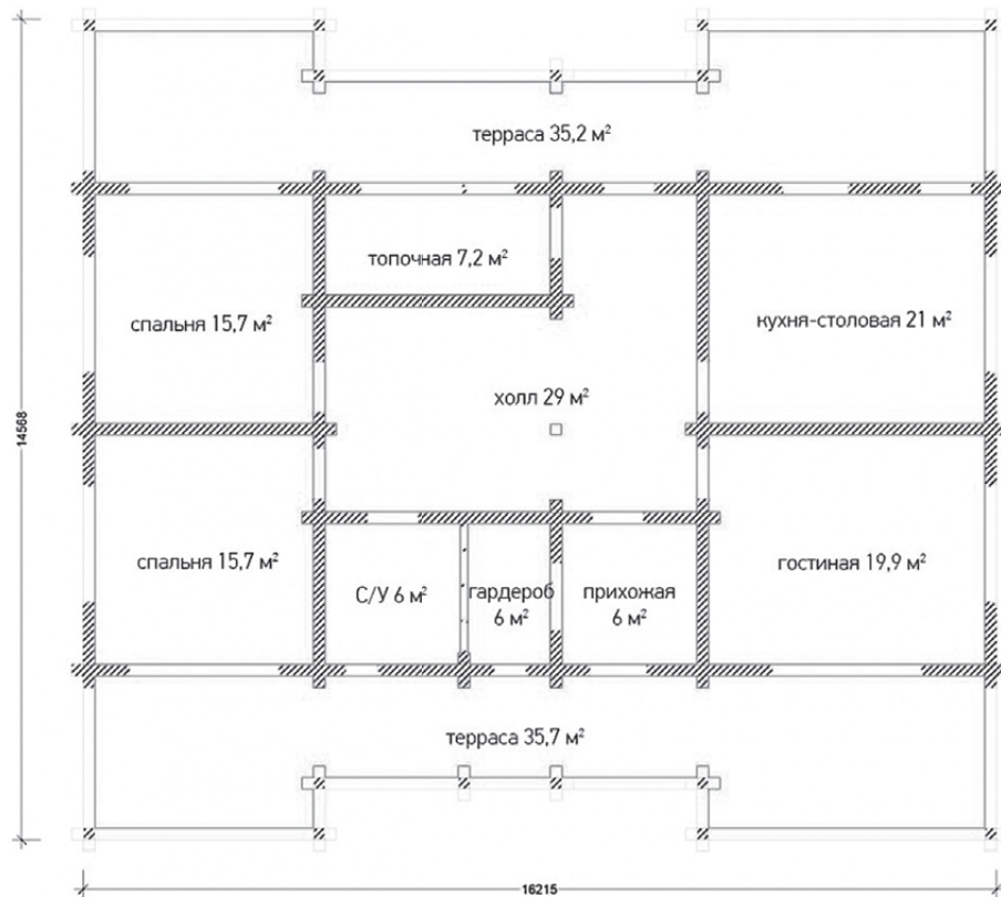
План 1 этажа
