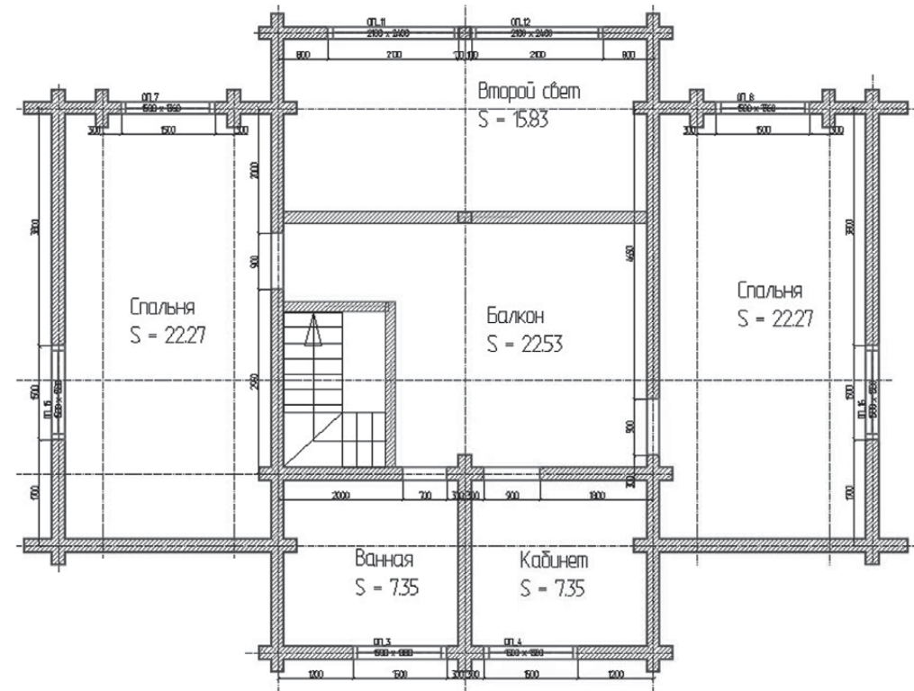
План 2 этажа
