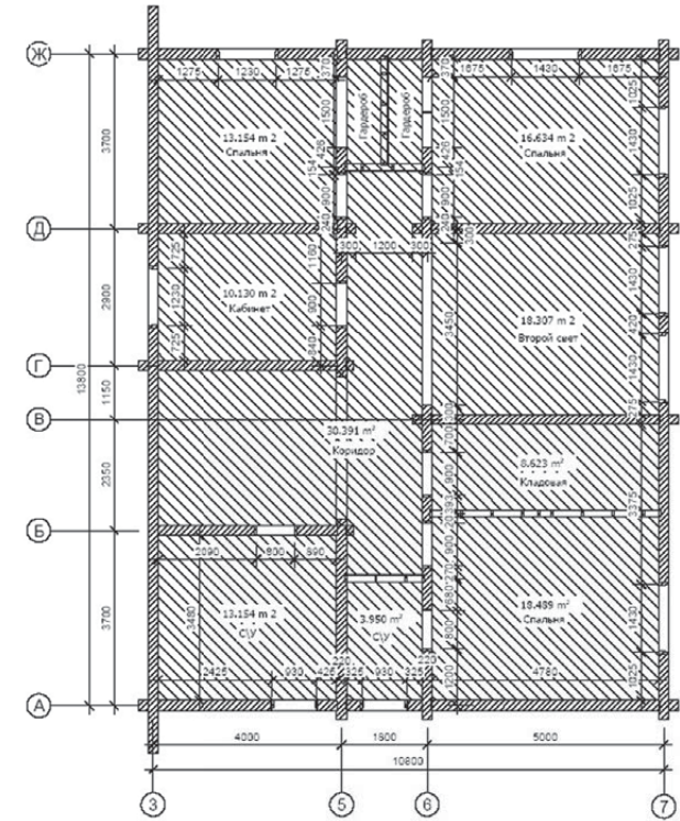
План 2 этажа
