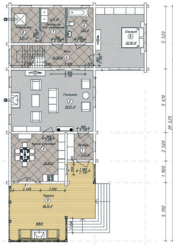
План 1 этажа
