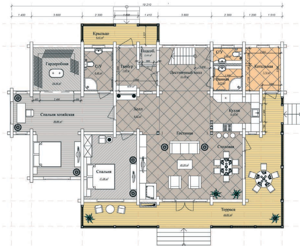
План 1 этажа
